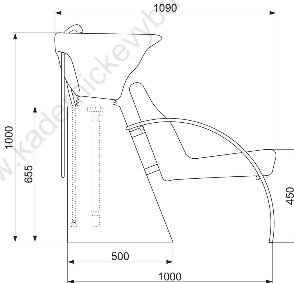
Boční pohled
