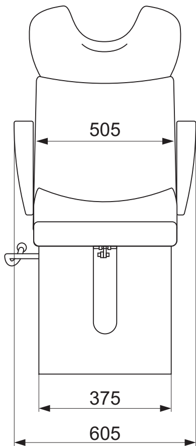
Čelní pohled
